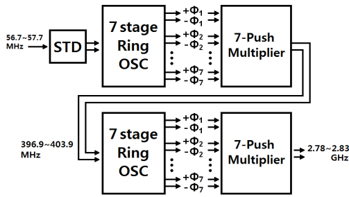
그림 1. 제안된 \times 49 체배기 블록 다이어그램 Fig. 1. Block diagram of the proposed \times 49 frequency multiplier.
