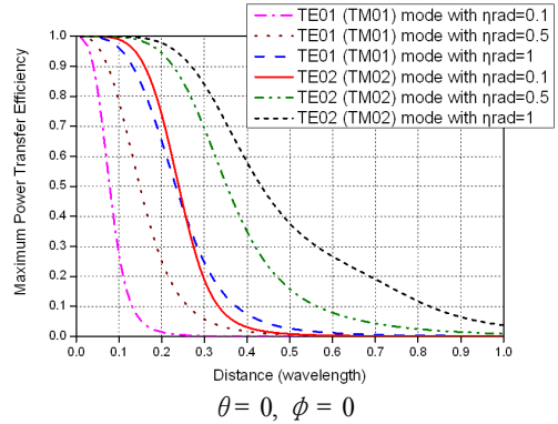
[그림 3] TE 01 (TM 01 ) 모드 안테나와 TE 02 (TM 02 ) 모드 안테나의 최대 파워 전송 효율
